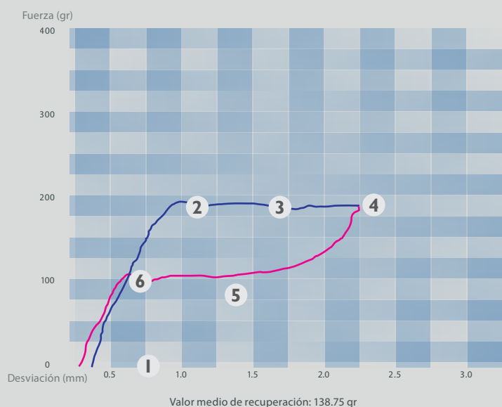
GRÁFICO DE HISTERESIS
